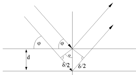
Abbildung 2: Reflexion von Röntgenstrahlen am Kristallgitter
